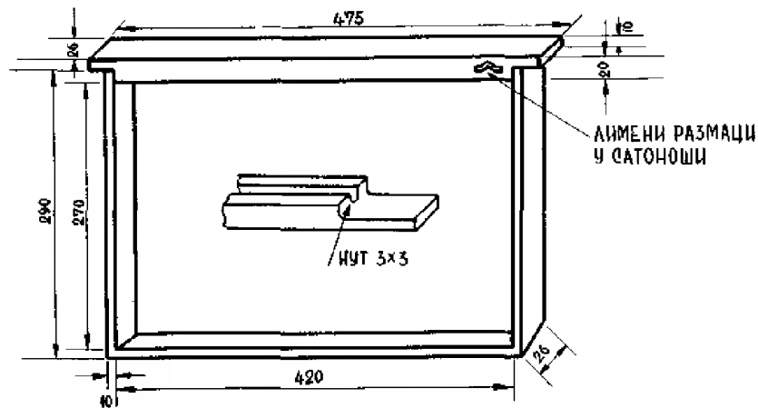
Плодишни оквир Дадан-Блатове кошнице (Мере изражене у mm)
